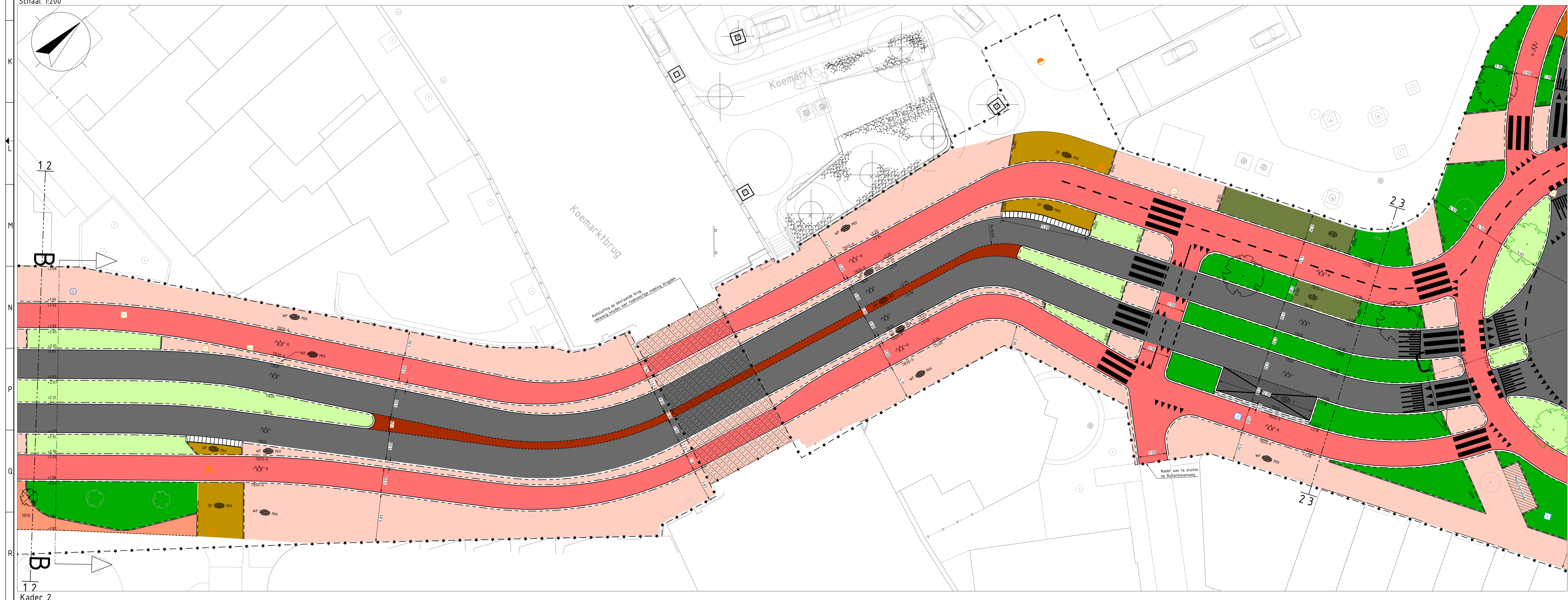
Kader 2 Schaal 1:200
