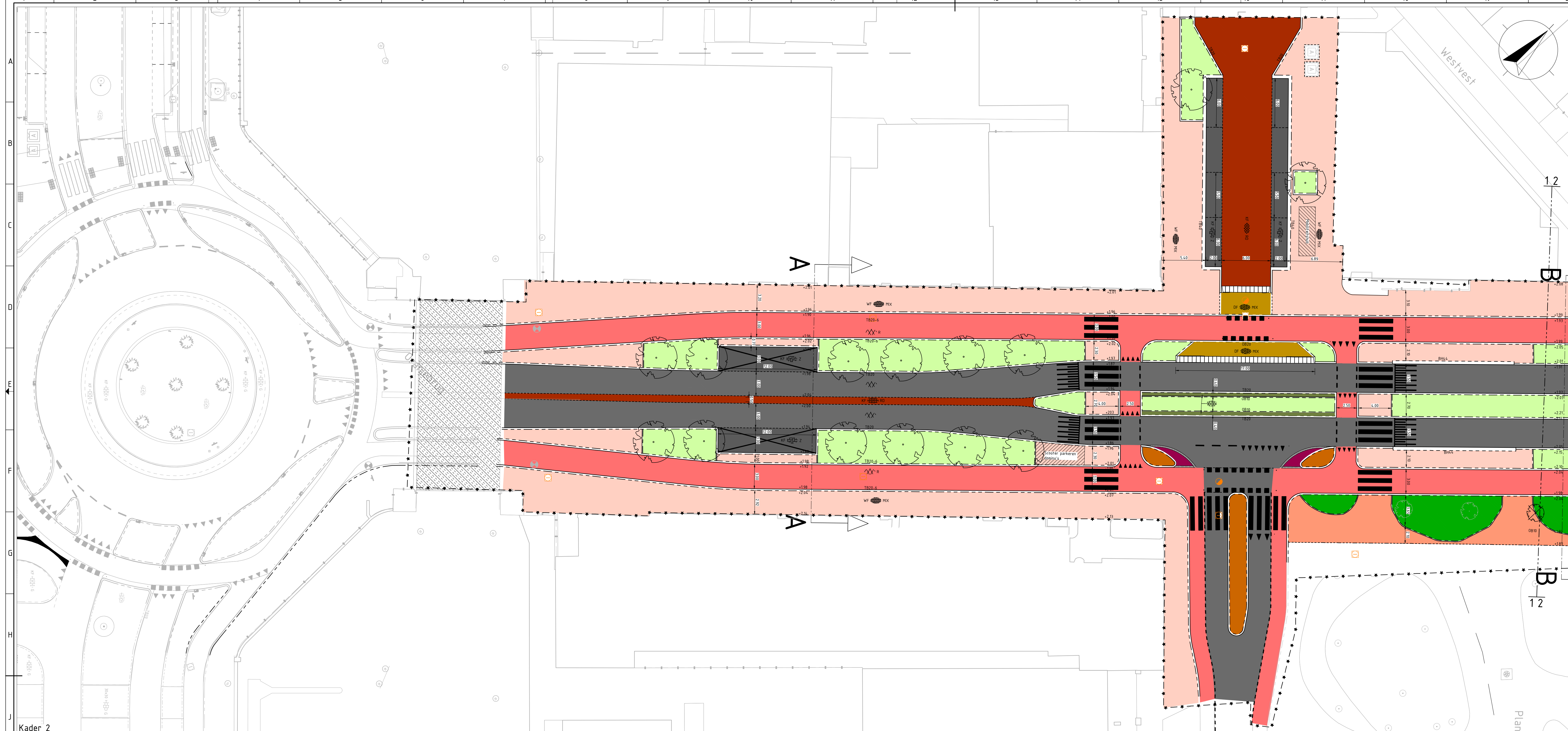
Kader 2 Schaal 1:200
