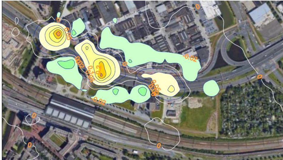
Figuur 7-28: Veranderingen in concentraties roet (EC) van lokale wegen als gevolg van de ontwikkeling Schieveste.
