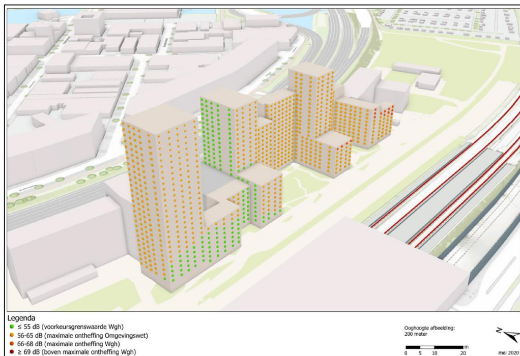
Figuur 10-8: Bollenkaart met geluidsbelasting ten gevolge van hoofdspoorwegen - realisatie fase 1
