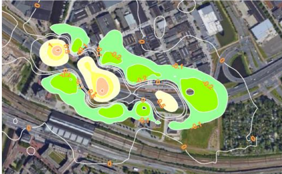
Figuur 7-27: Veranderingen in concentraties PM_{10} als gevolg van de ontwikkeling Schieveste.
