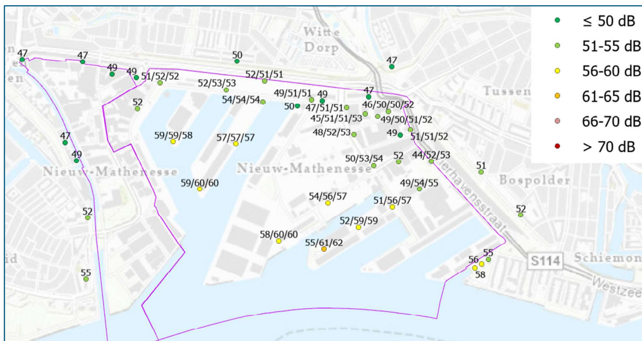
Figuur 4.6: Geluidsbelasting in L_{den} als gevolg van het scheepvaartlawaai in de referentiesituatie
