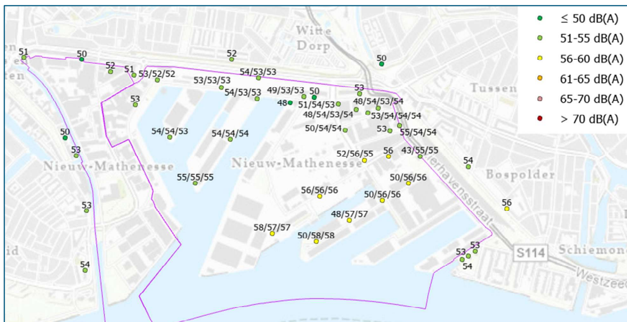
Figuur 4.2: Geluidsbelasting in Letmaai als gevolg van het gezoneerde industrielaawaai WEH in de referentiesituatie
