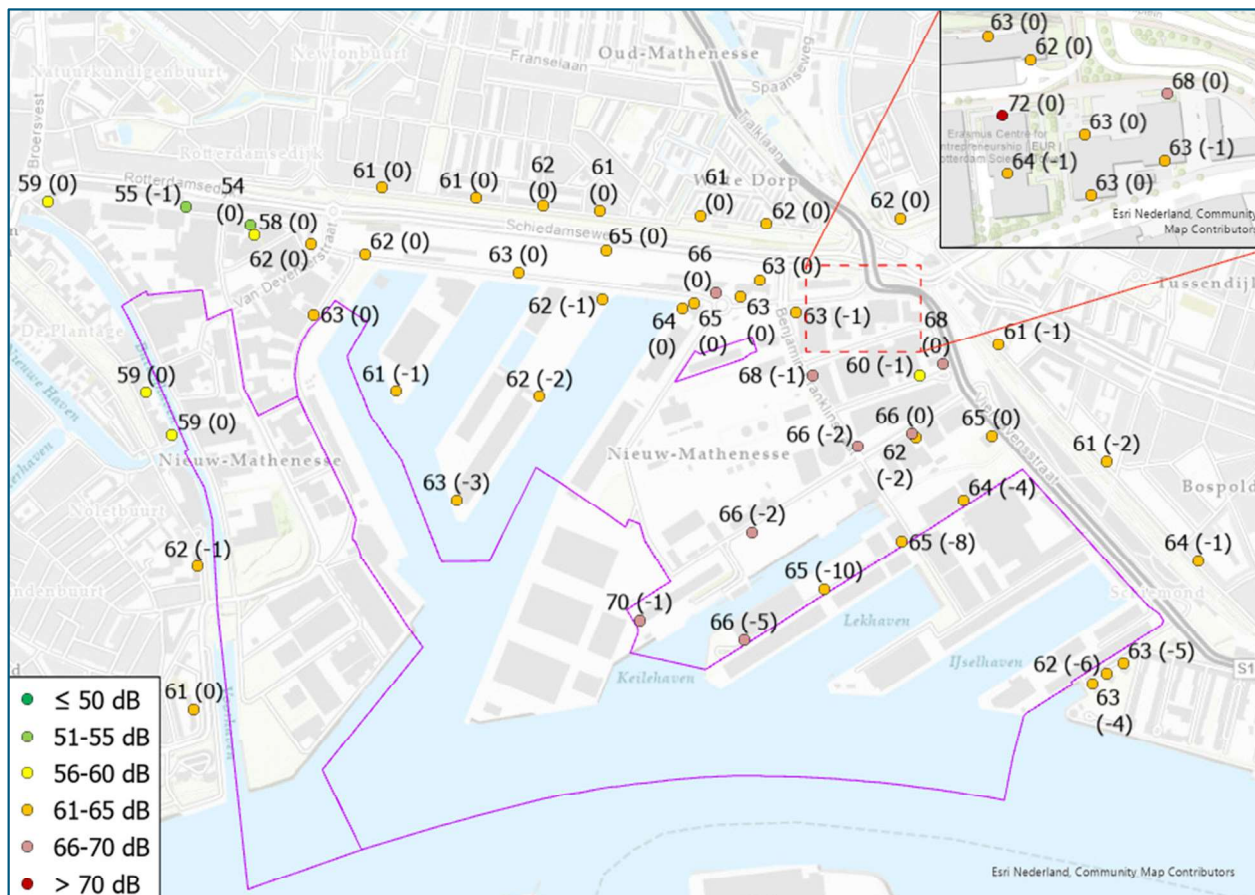
Figuur 6.4: Cumulatieve geluidsbelasting L_{cum} in de toekomstsituatie na toepassen nestgeluidmaatregelen toekomtperspectief
