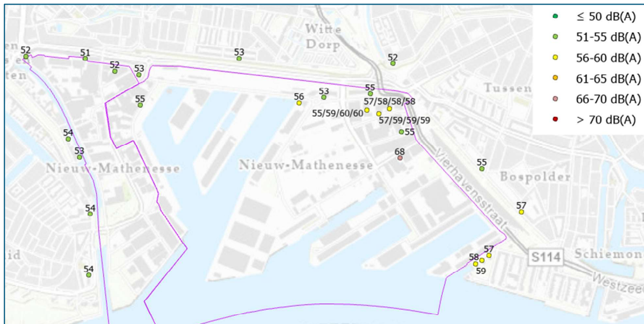
Figuur 3.3: Geluidsbelasting in Letmaal als gevolg van het huidige gezoneerde industrielawaai HNOF en WEH
