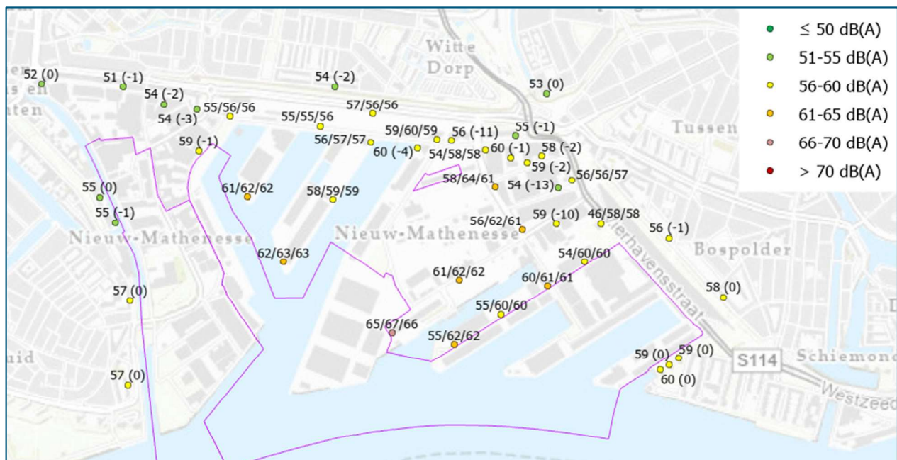
Figuur 5.4: Totale geluidsbelasting in L_{etmaal} als gevolg van al het industrielawaai in de toekomstsituatie
