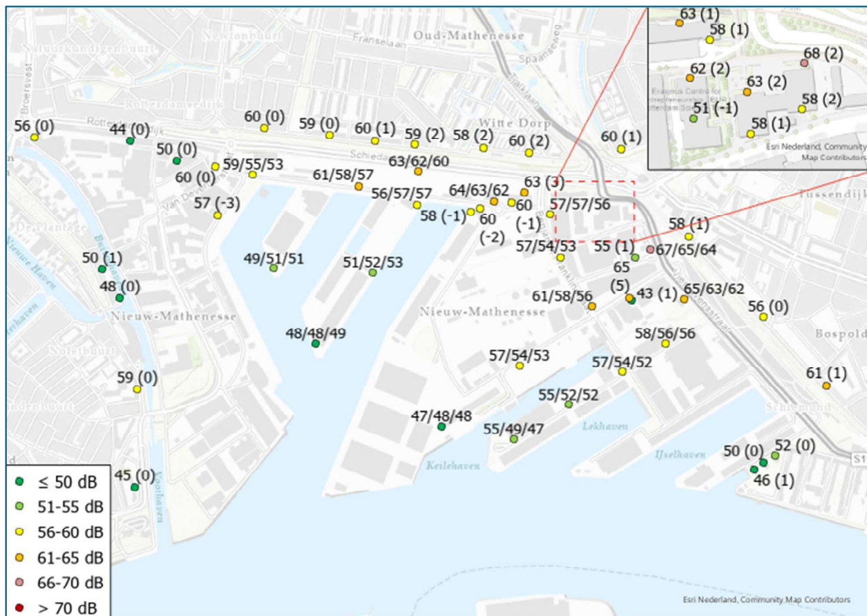
Figuur 5.6: Geluidsbelasting in L_{den} als gevolg van het wegverkeerslawaaï variant 4, excl. aftrek art. 110g Wgh.
